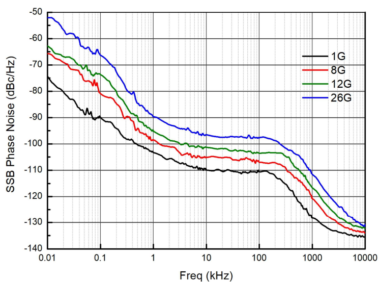
单边带相位噪声
